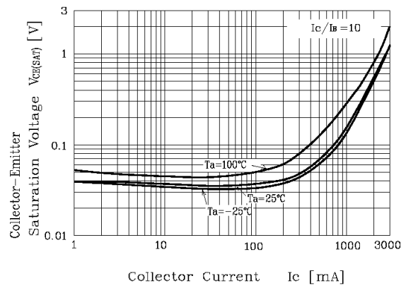
Fig. 4 V_{CE(sat)} - I_C
